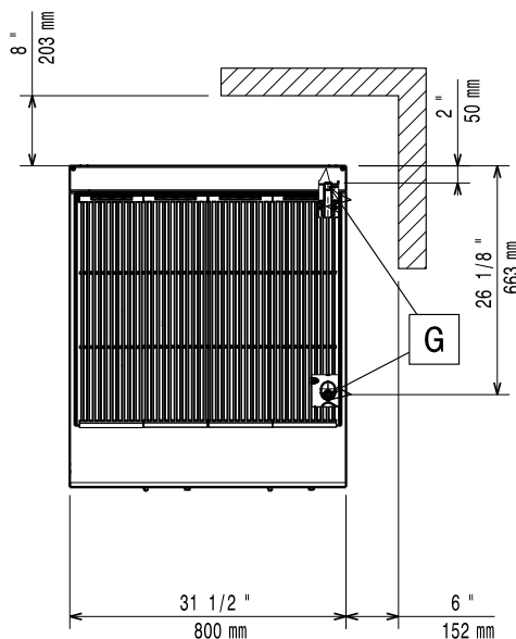
Boven aanzicht
